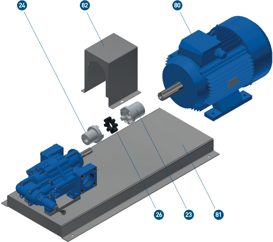
Fig. 531 – MBM-MBMC
