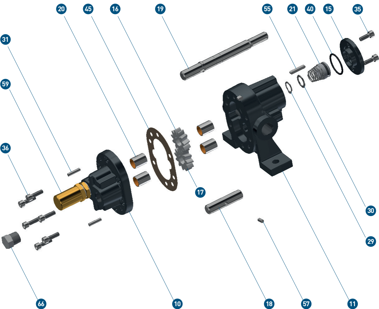
Fig. 521 - B5-40; BC10-25
